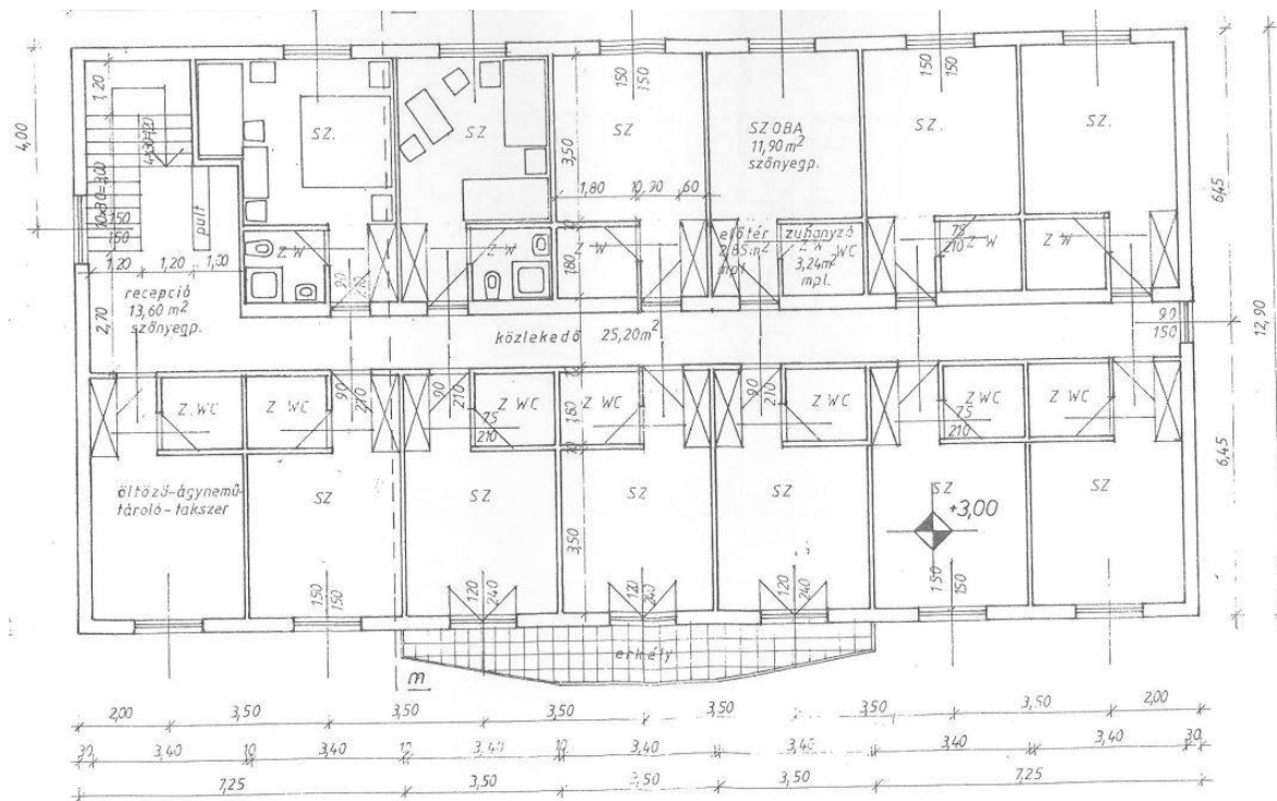
emeleti alaprajz
