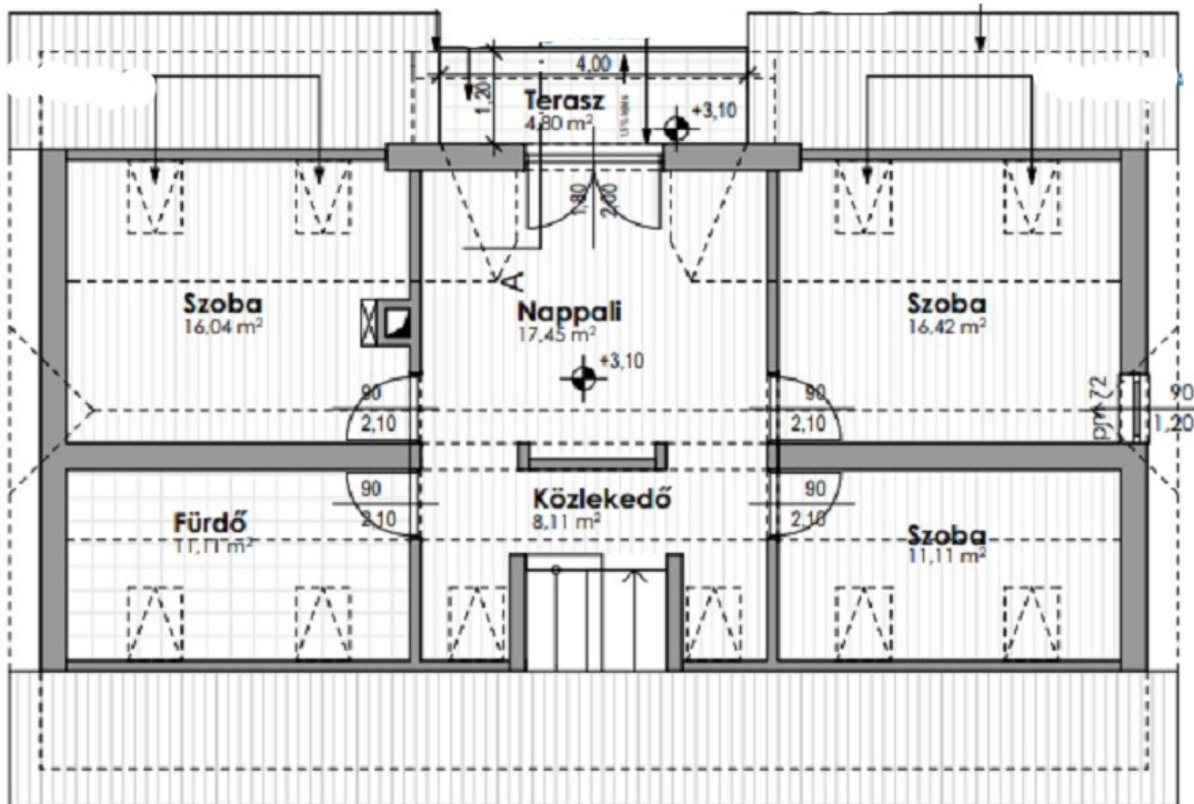
Tetőtér alaprajza
