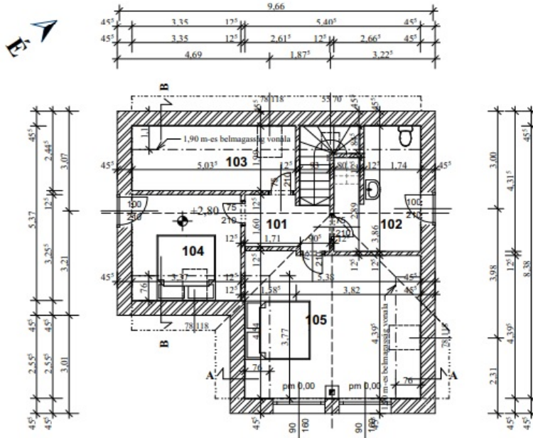
TERVEZETT TETŐTÉRI ALAPRAJZ M = 1 : 100
