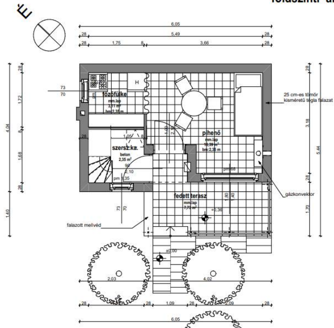
földszinti alaprajz
