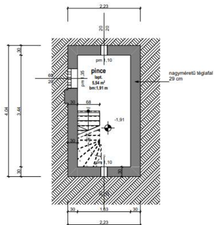
pincszinti alaprajz
