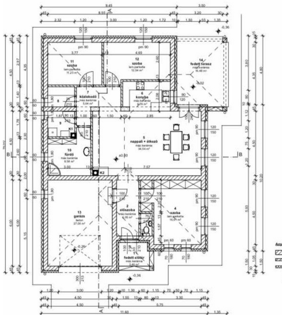
Alaprajz M1:100
