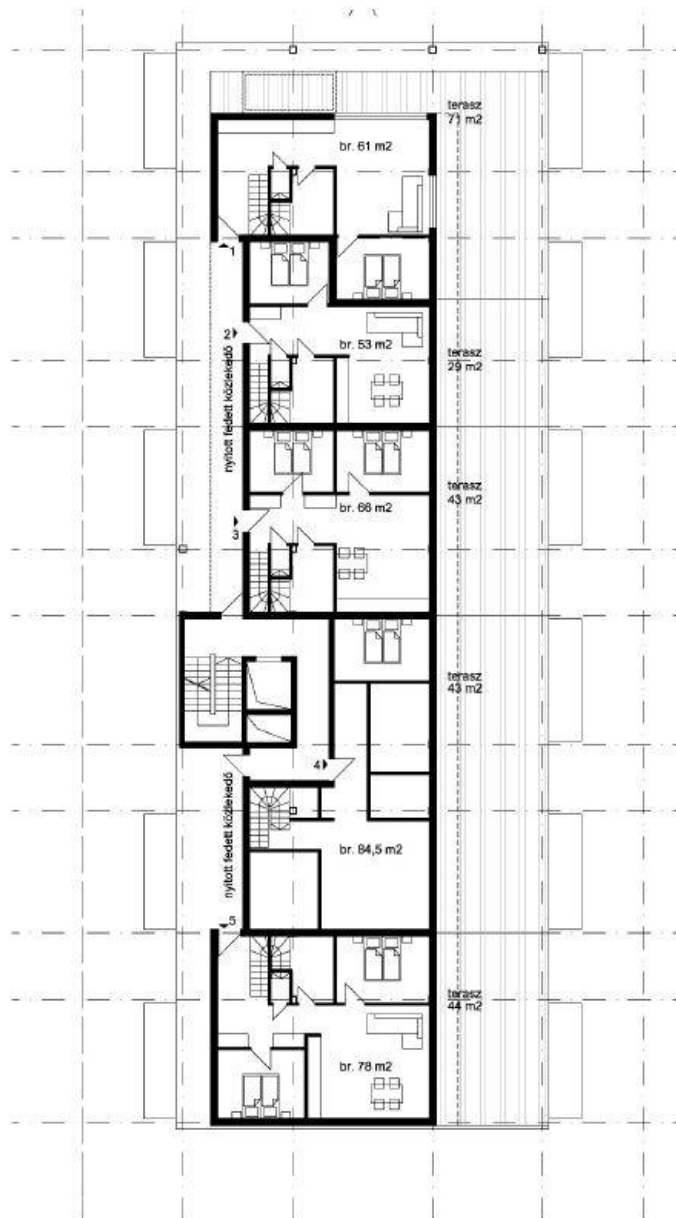
2. EMELET ALAPRAJZ
