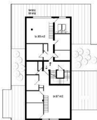
2. EMELETI ALAPRAJZ
