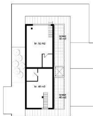
3. EMELETI ALAPRAJZ
