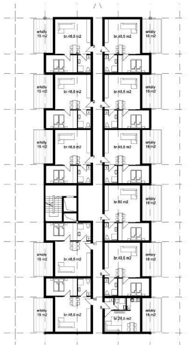
EMELETI ALAPRAJZ
