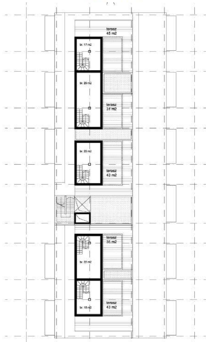
3. EMELETI ALAPRAJZ
